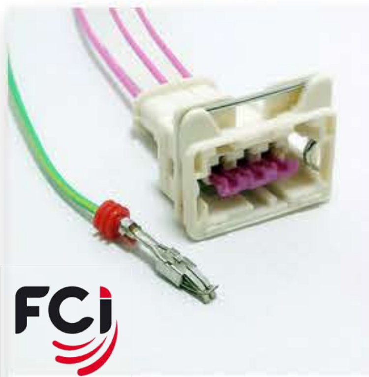
خانه 2 سوکت ترمینال وسیل خورده 3 F.C.I خانه
